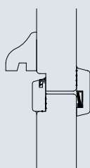
doorsnede duodeling met dubbele tochtwering
