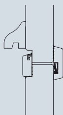
doorsnede duodeling met dubbele tochtwering
